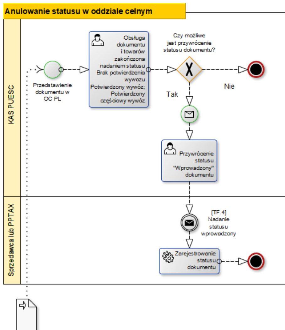
Rysunek 10 Schemat procesu anulowania statusu w oddziale celnym
