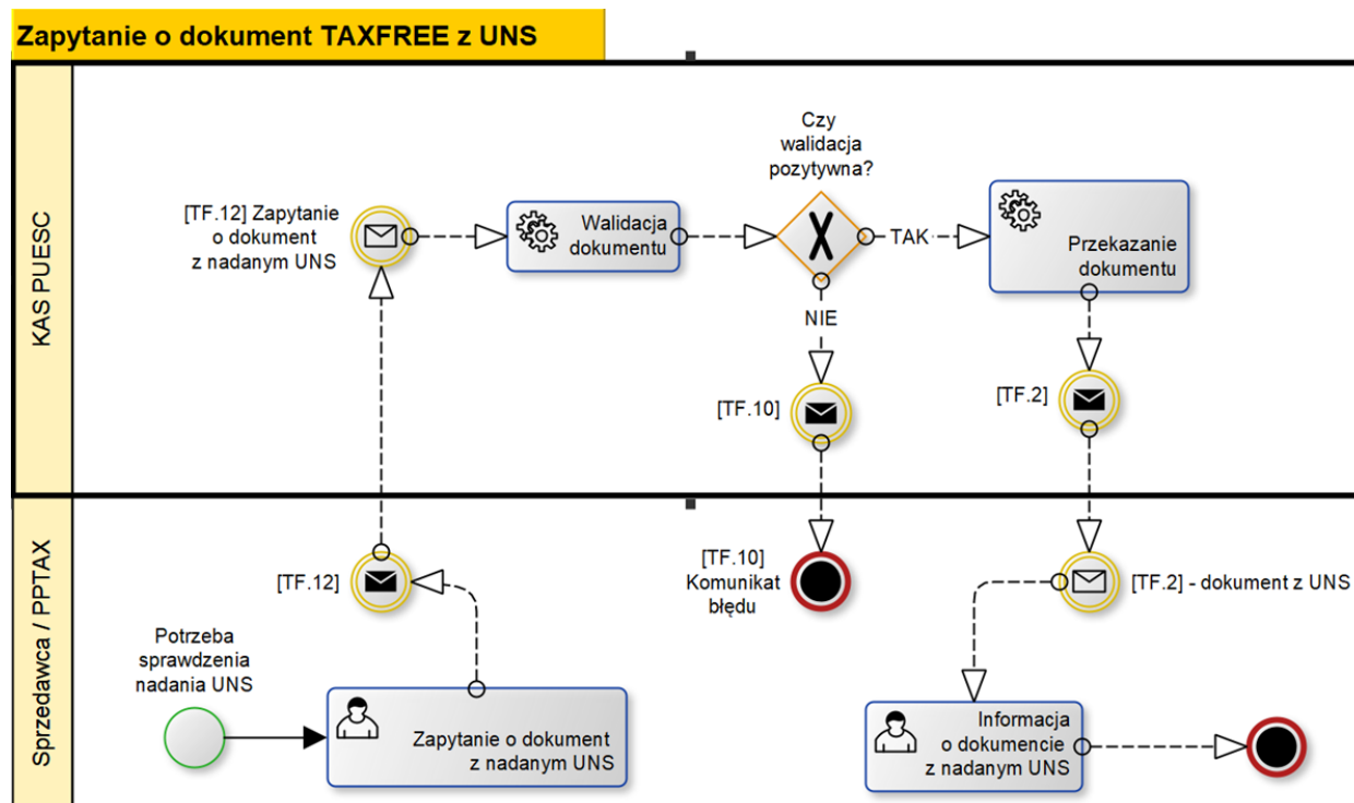
Rysunek 9 Schemat procesu zapytania o dokument TAXFREE z UNS
