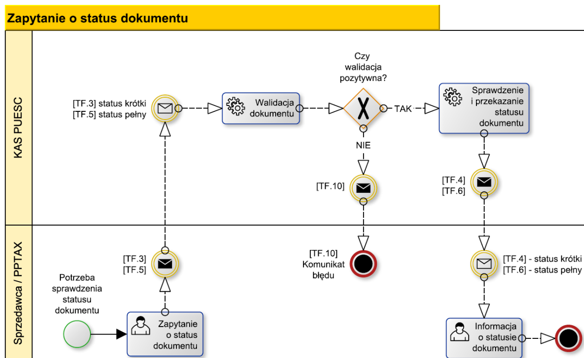
Rysunek 6 Schemat procesu zapytania o status dokumentu
