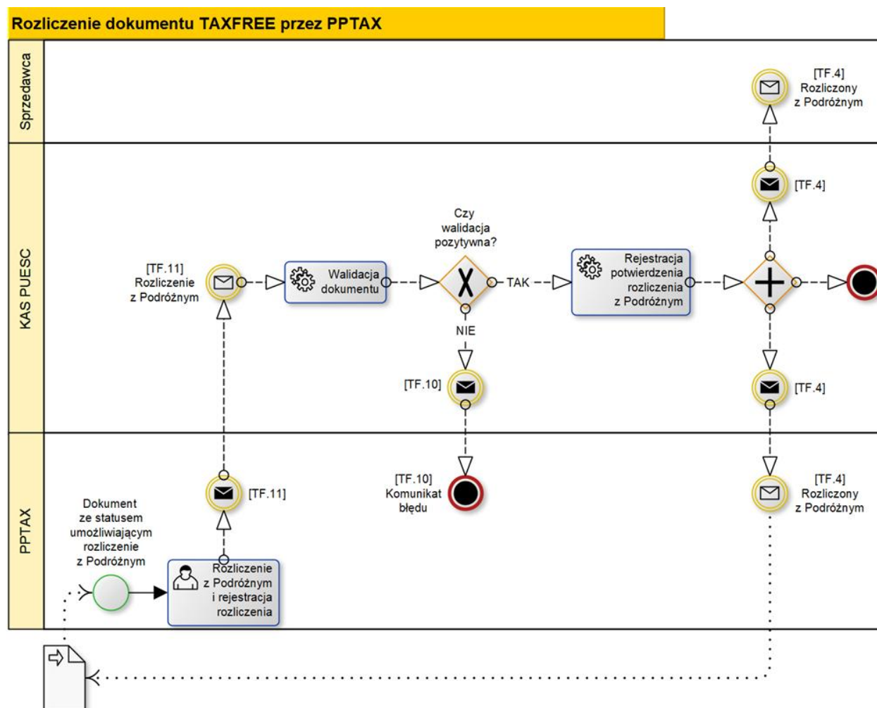
Rysunek 5 Schemat procesu rozliczenia dokumentu TAXFREE przez PPTAX
