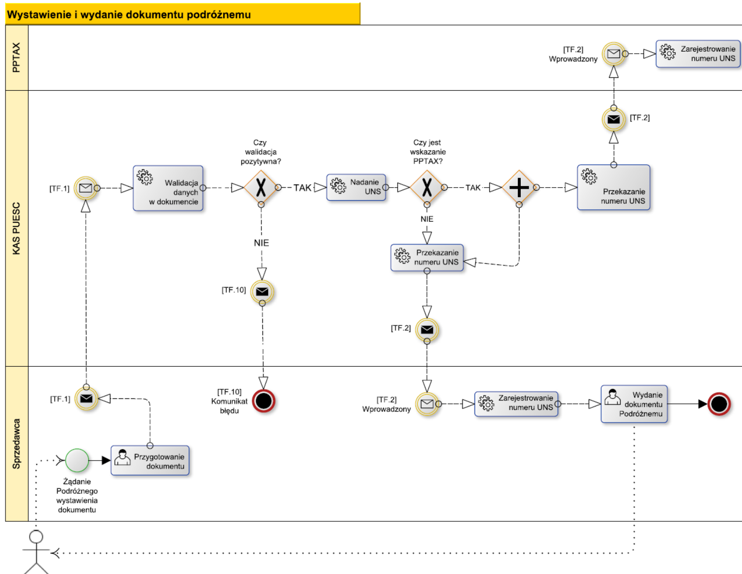
Rysunek 2 Schemat procesu wystawienia i wydania dokumentu podróznego
