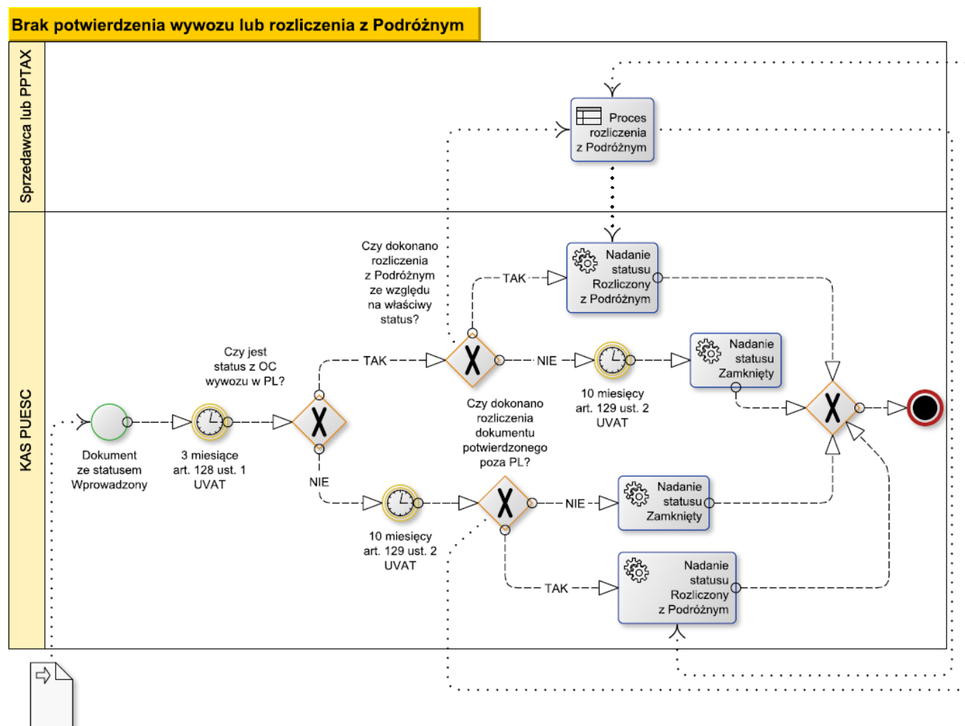
Rysunek 8 Schemat procesu unieważnienia dokumentu
