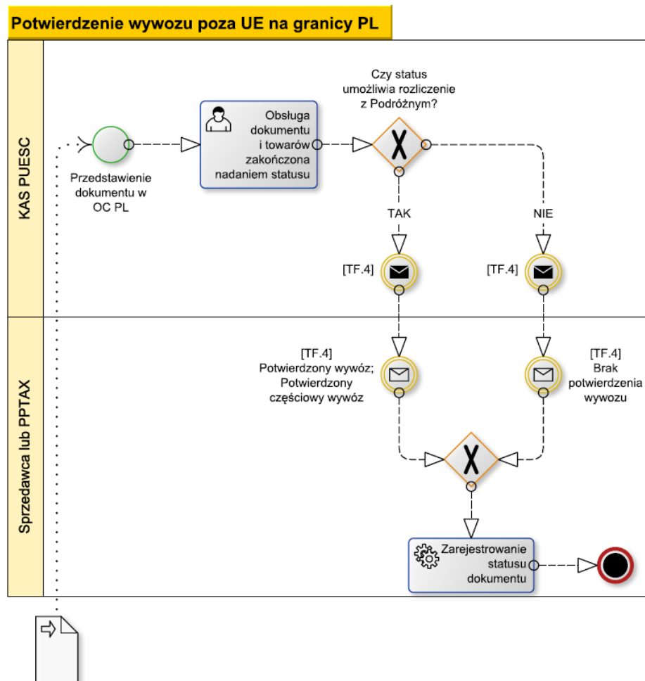
Rysunek 3 Schemat procesu potwierdzenia wywozu poza UE na granicy PL
